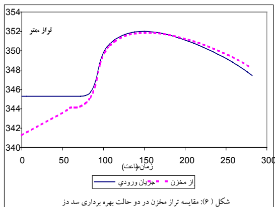
شکل (۶): مقایسه تراز مخزن در دو حالت بهره برداری سد دز
