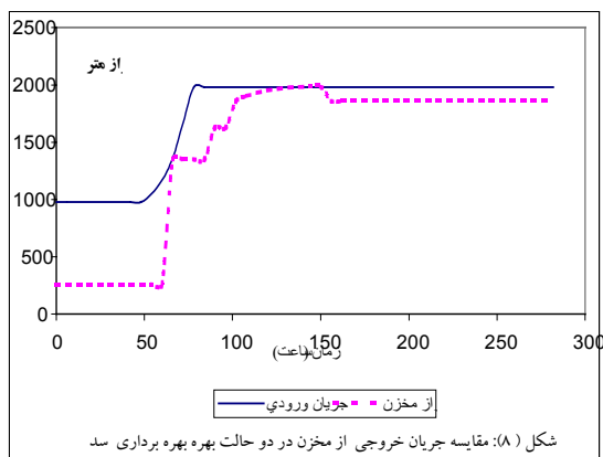
شکل (۸): مقایسه جریان خروجی از مخزن در دو حالت بهره برداری سد
